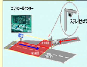
【逆走検知システム】
