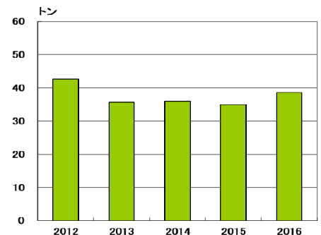
事業系一般廃棄物排出量の推移
