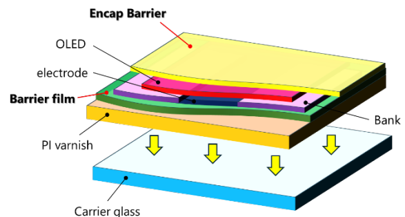
▼試作したフレキシブルOLEDの構成図
